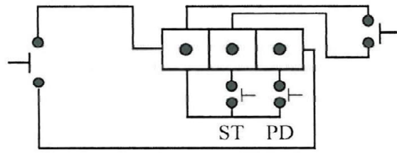
۱- استارت دولنگه
