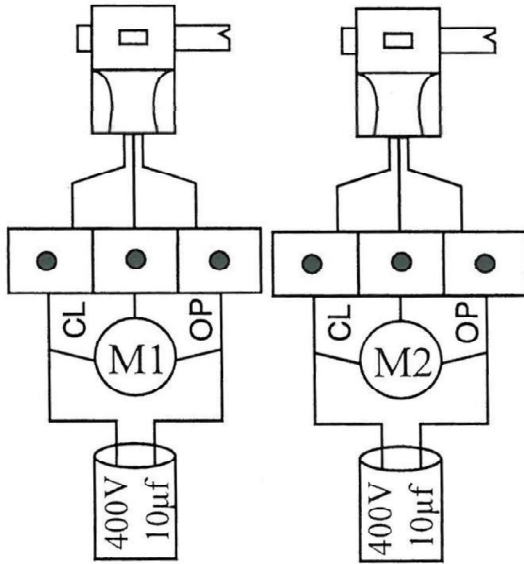
۶- لیمیت سوئیچ
