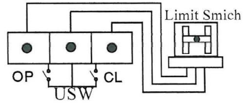
۵- قفل برقی
